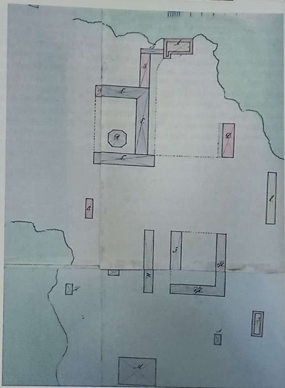
План усадьбы Г.Н. Вельяминова в с. Никольское, 1898 г. ЦГАМ
